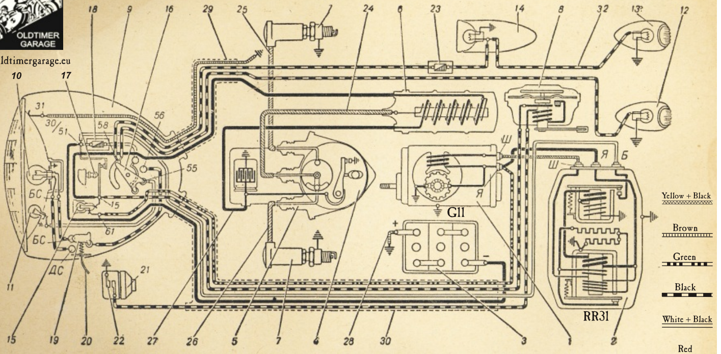
Фиг. 69а. Схемы электрооборудования мотоцикла М-72:
